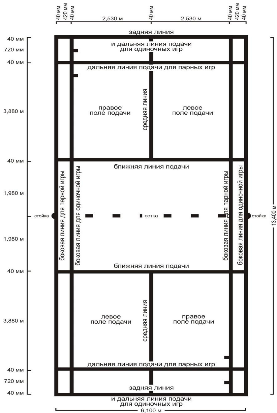
Рис. 1. Разметка корта для парной и одиночной игры.
