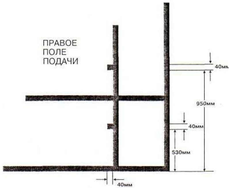
Рис. 2. Контрольные метки для тестирования воланов.
